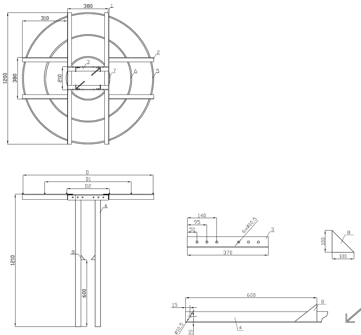
Фиг. 1 - Метални платформи за повдигане на щъркелови гнезда върху стоманобетонни стълбове.
